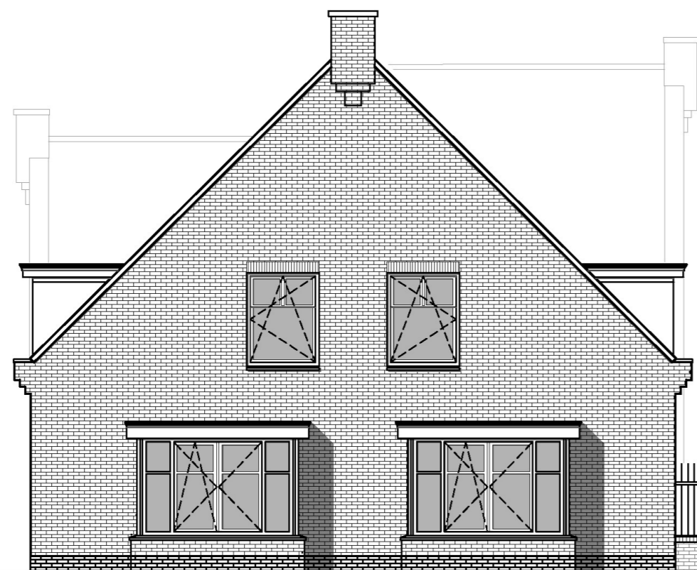
kopgevel - kloosterzijde -
