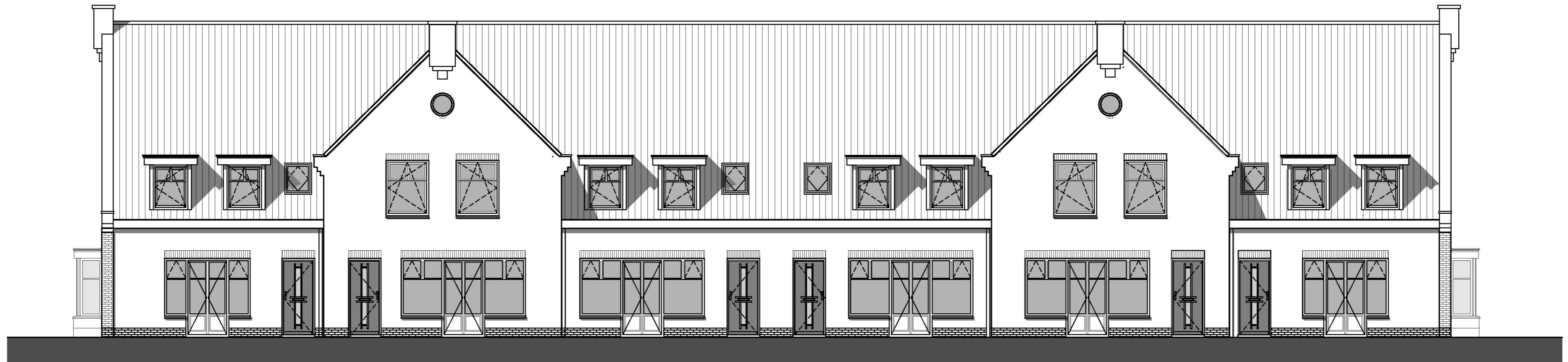
Gevel hofwoningen
