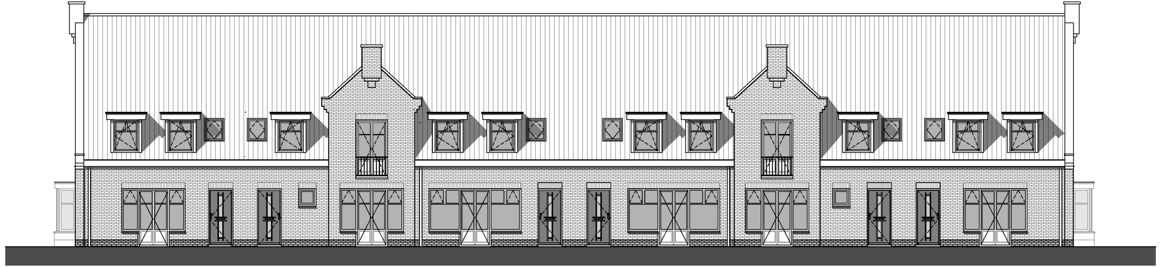
Gevel tuinwoningen
