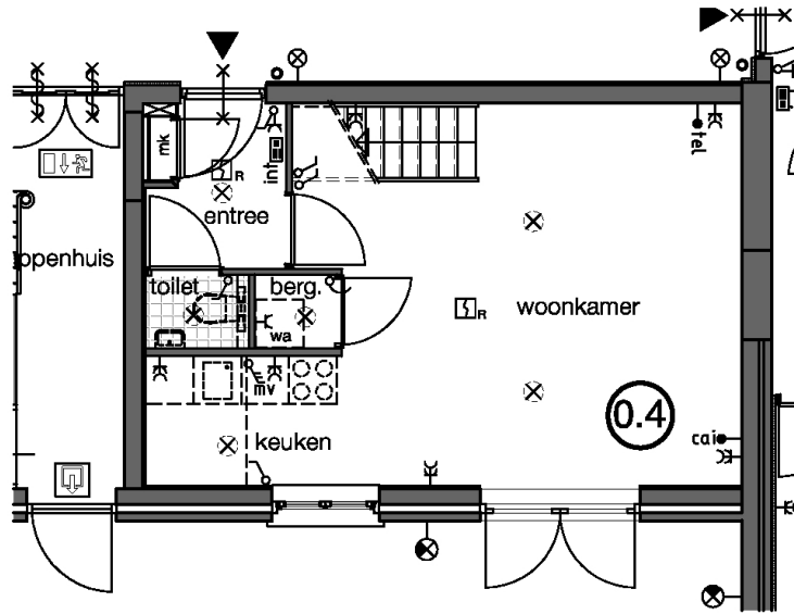
begane grond
