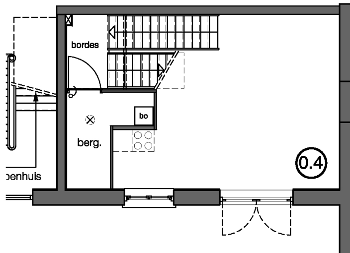
tussenverdieping
