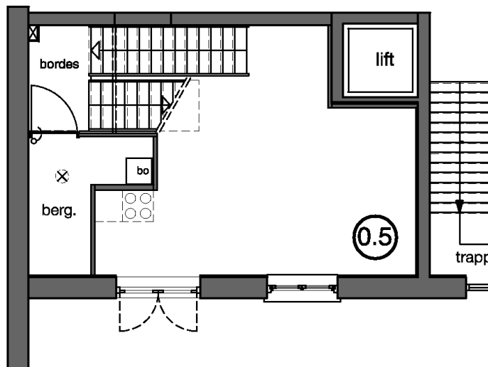
tussenverdieping
