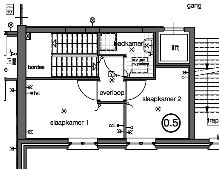
eerste verdieping
