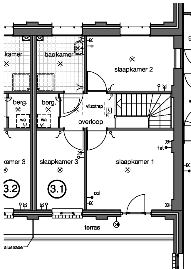
eerste verdieping
