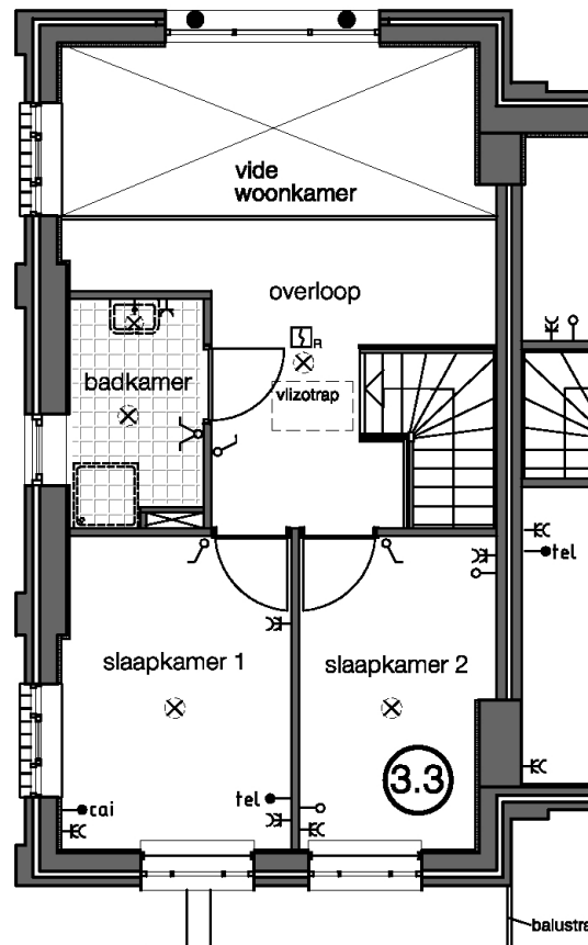
eerste verdieping
