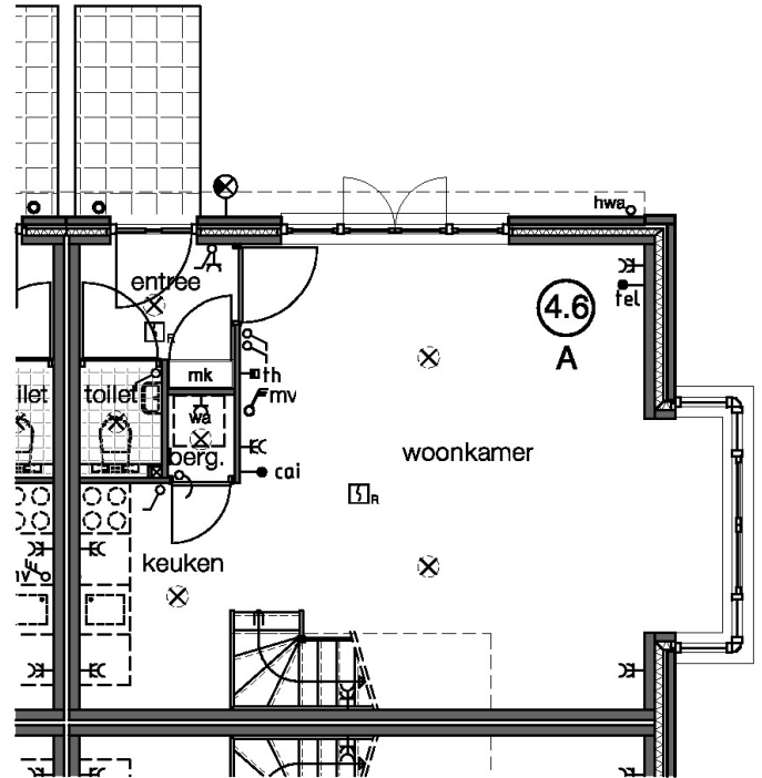
begane grond
