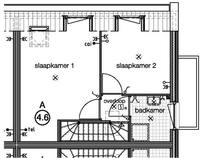
eerste verdieping
