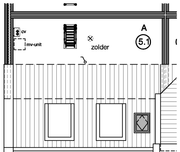
2 tweede verdieping
