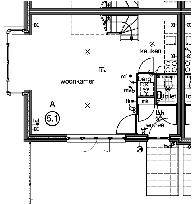
begane grond
