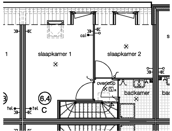
eerste verdieping
