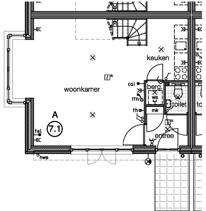
begane grond
