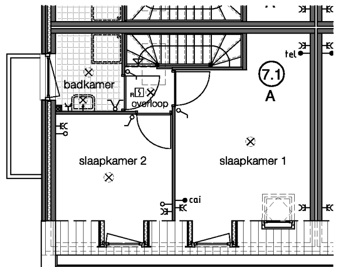
eerste verdieping
