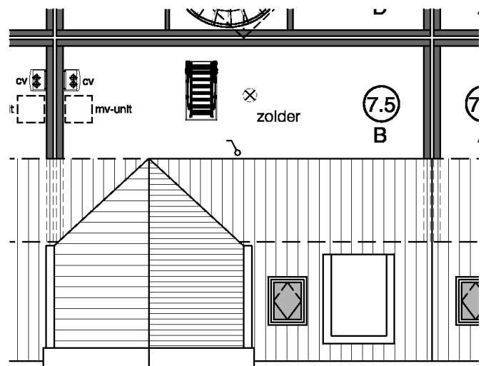
tweede verdieping
