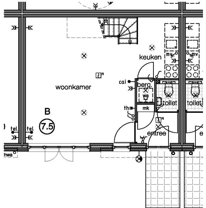
begane grond
