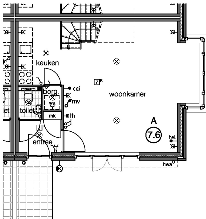
begane grond
