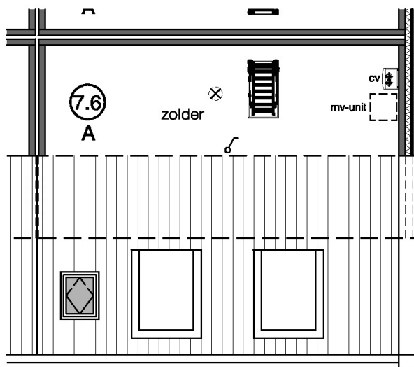
tweede verdieping
